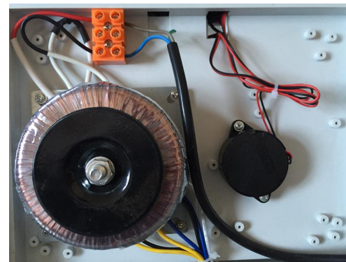
变压器安装示意图
